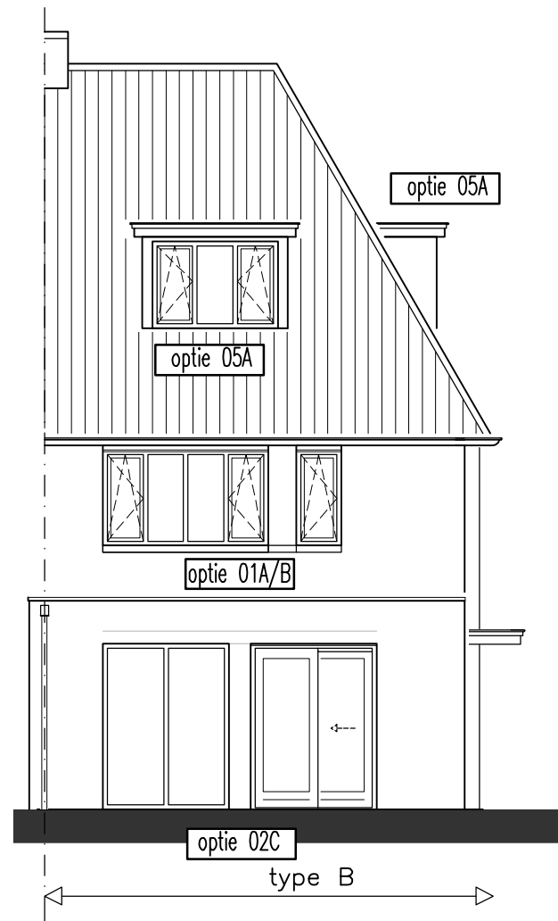
ACHTERGEVEL
