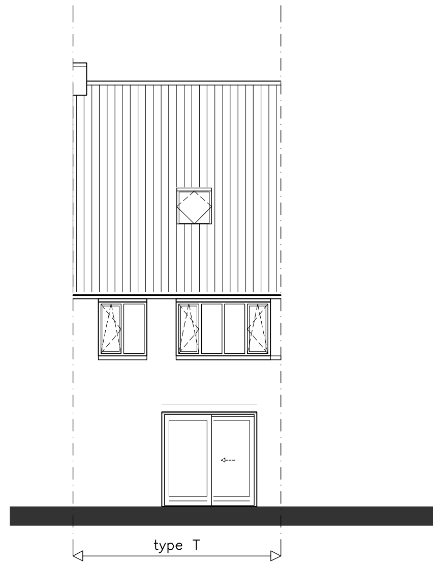
ACHTERGEVEL
