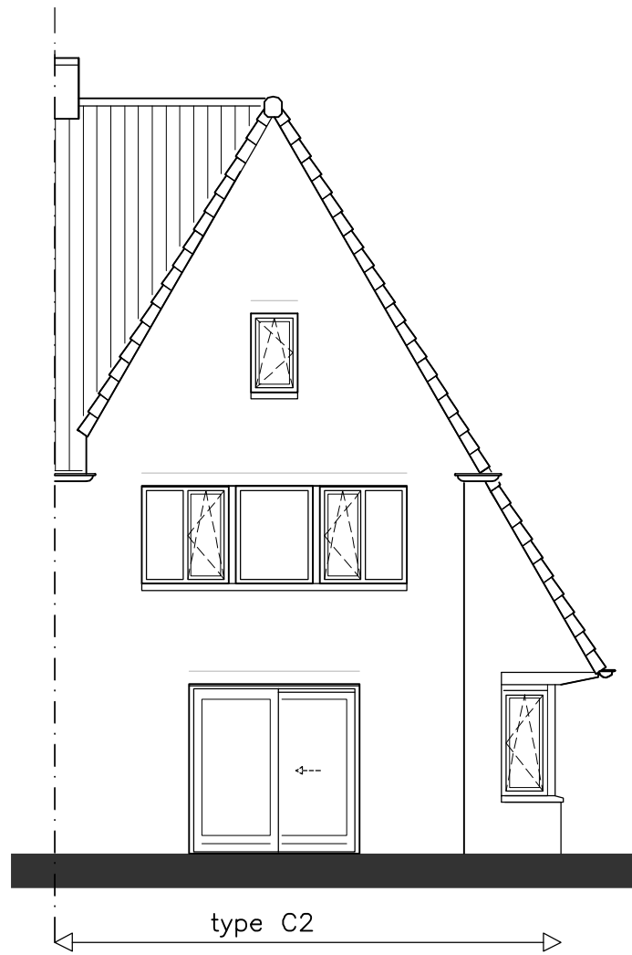
ACHTERGEVEL
