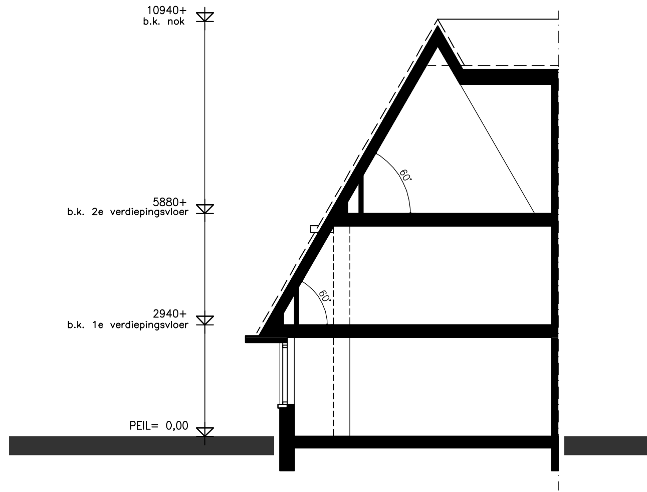
DOORSNEDE
