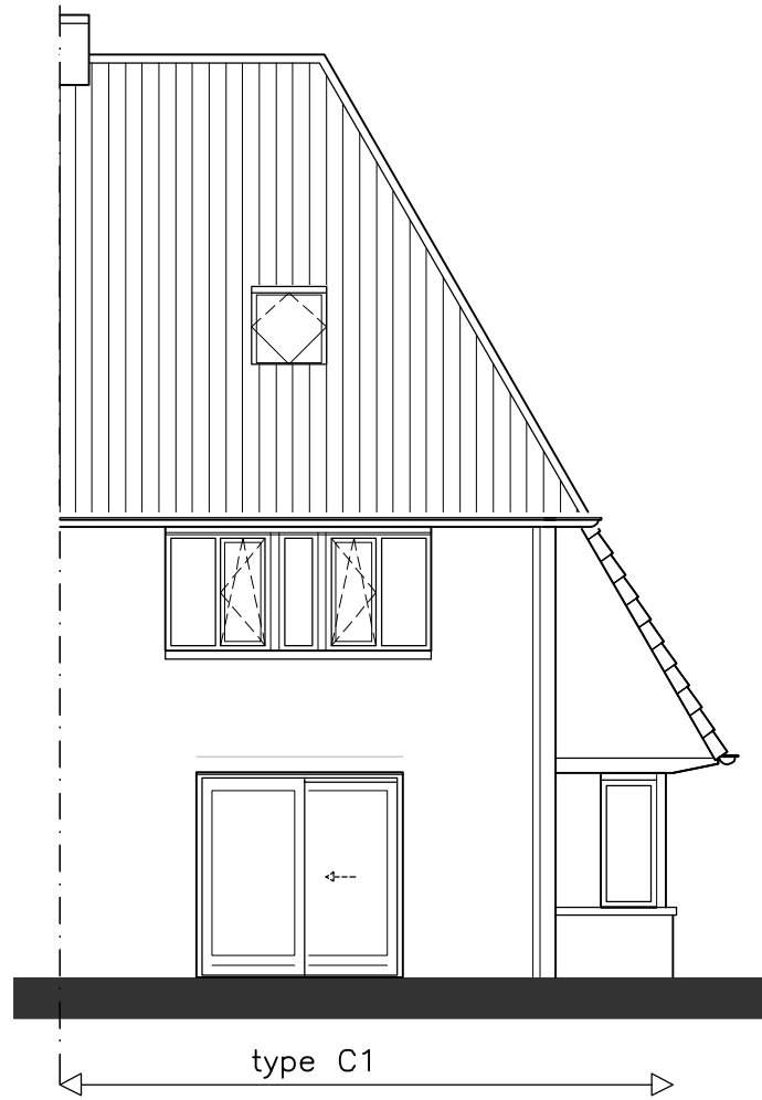
ACHTERGEVEL
