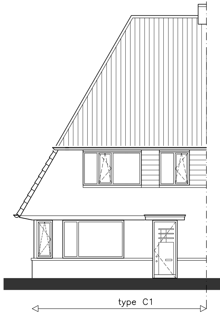
VOORGEVEL
