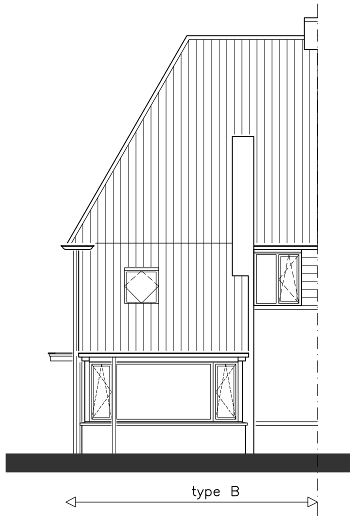
VOORGEVEL
