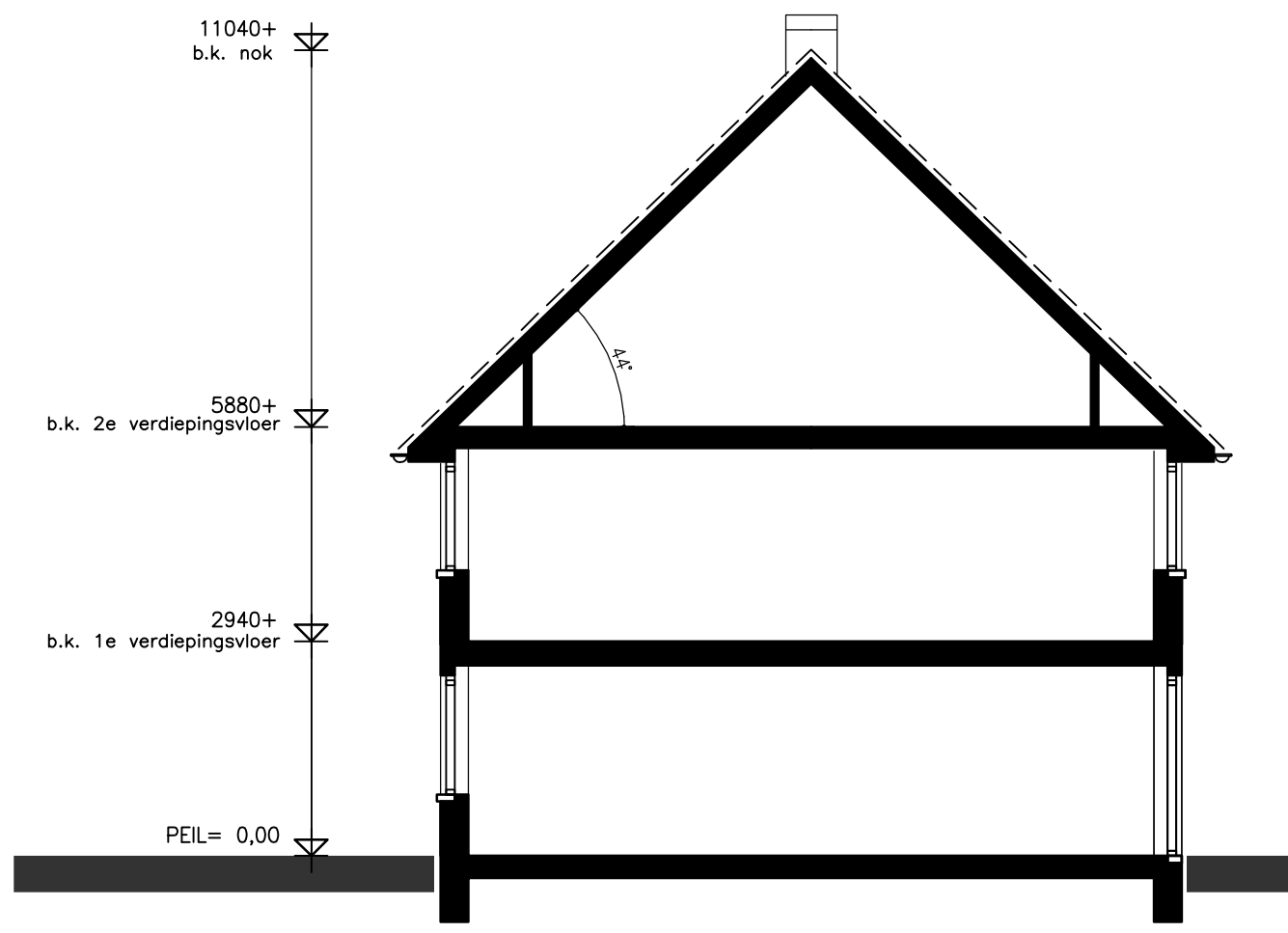
DOORSNEDE
