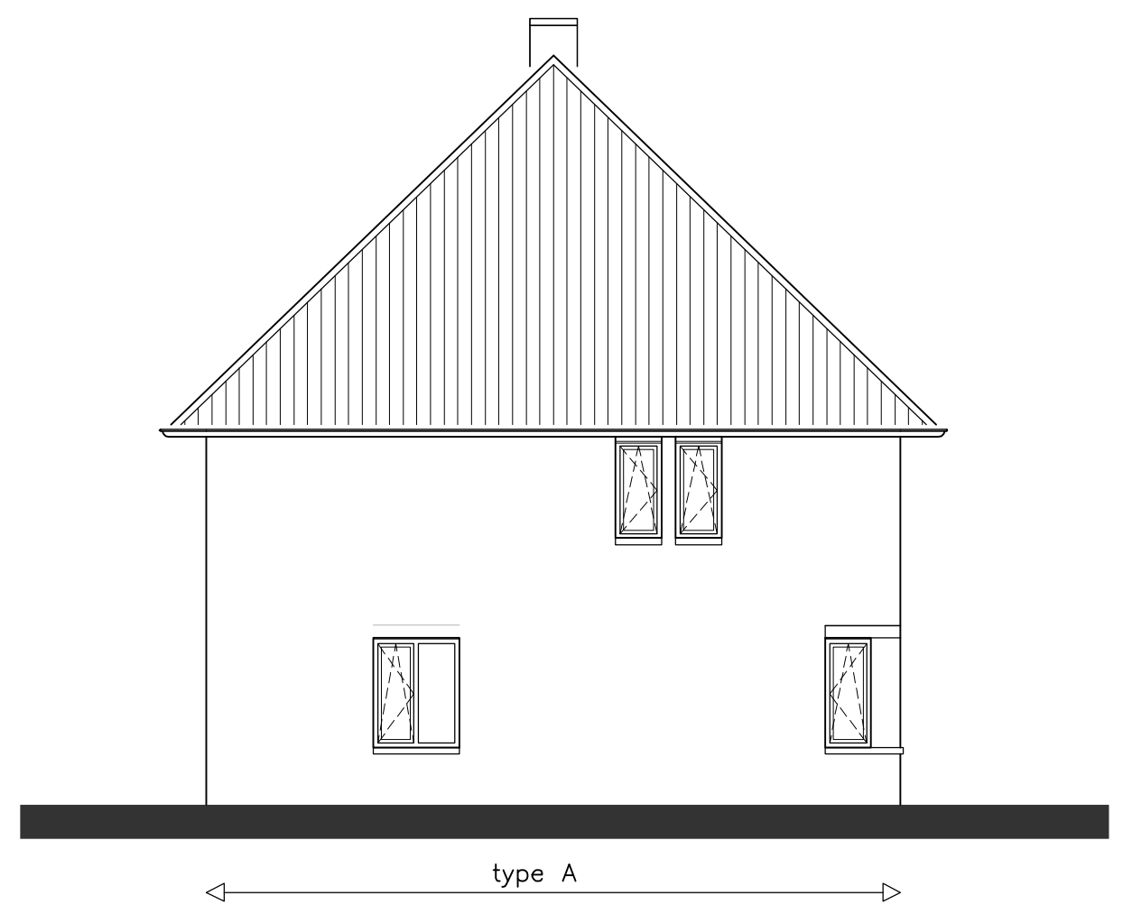
ZIJGEVEL
