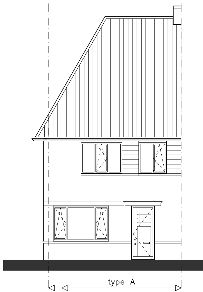
VOORGEVEL
