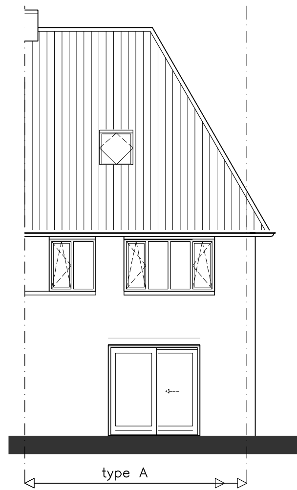
ACHTERGEVEL
